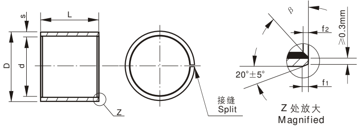
内外倒角
